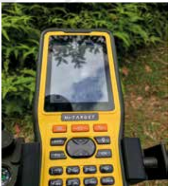
83.10. Zestaw RTK (kontroler i odbiornik) (wersja dwuelementowa- kontroler i odbiornik, lub zintegrowana)
